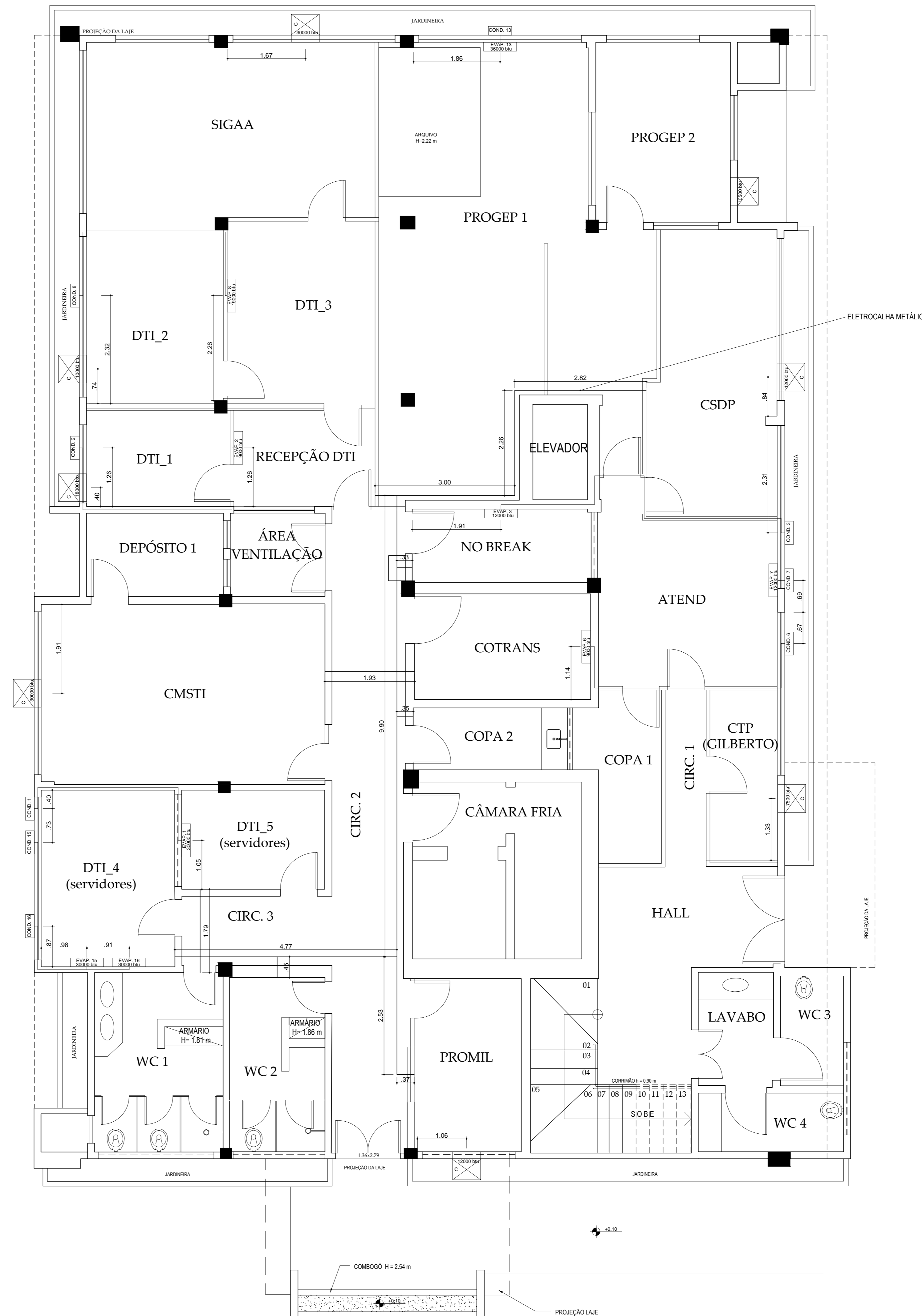
LOCAÇÃO AR-CONDICIONADO E ELETROCALHA PAV. TÉRREO (REFEITÓRIO) ESC.: 1/50
